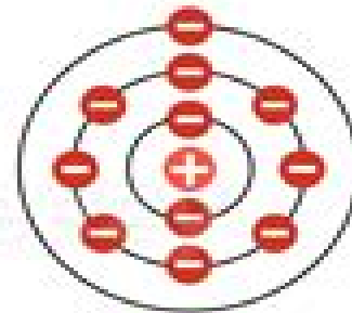
1913 Niels Bohr
