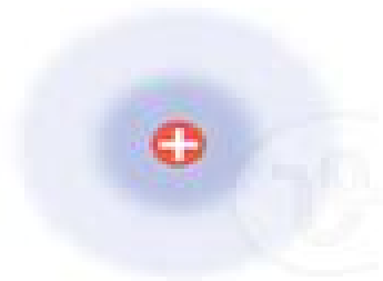
1926 Erwin Schrödinger
