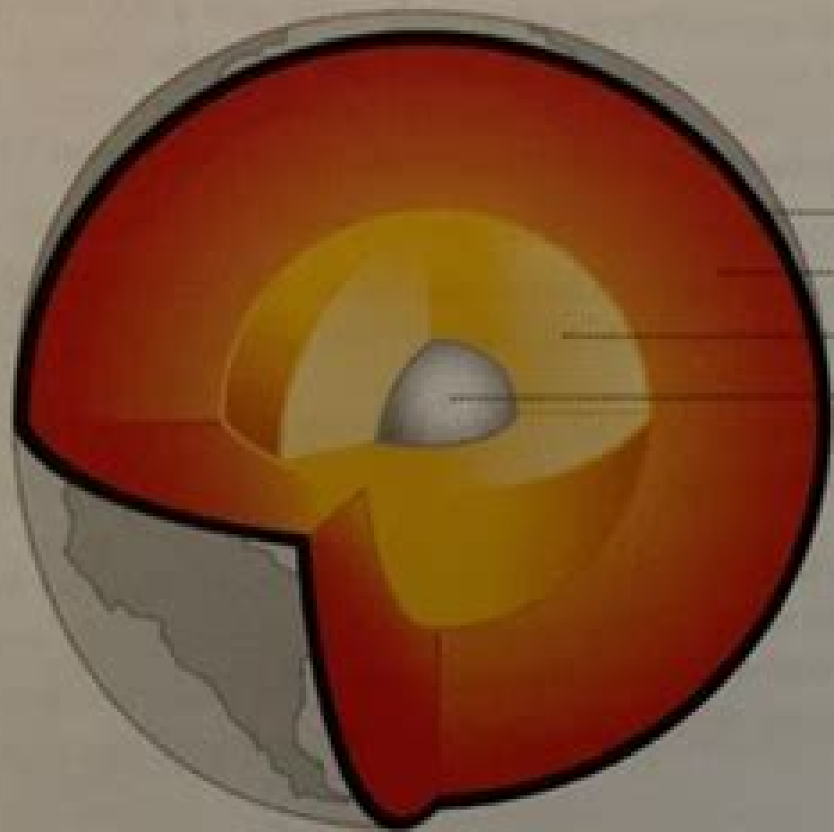
[Abb. 1-1] Schalenbau der Erde
