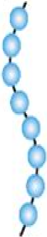
Linear
