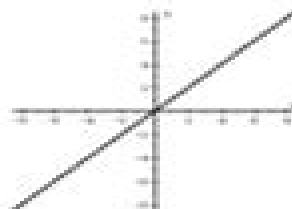
Linear
