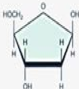
DEOXYRIBOSE
