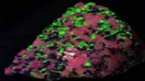
Calcite-Willemite-Franklinite
