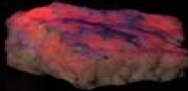
Quartz-Calcite-Rhodonite
