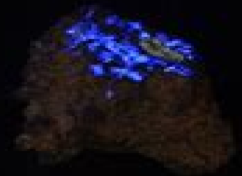
Manganese
