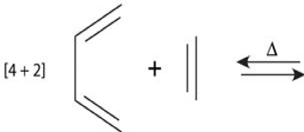
Butadiene
