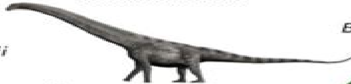
Ruyangosaurus giganteus
