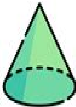
cone
