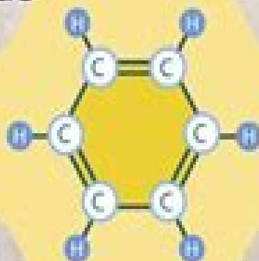
benzene
