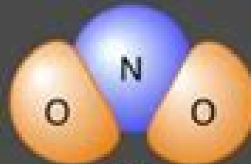
NO_2 nitrogen dioxide
